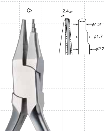
▲ 60-305 ループ フォーミング プライヤー LOOP FORMING PLIER CODE NO.63050 全長：約 125mm Wires up to.022" (0.55mm)
