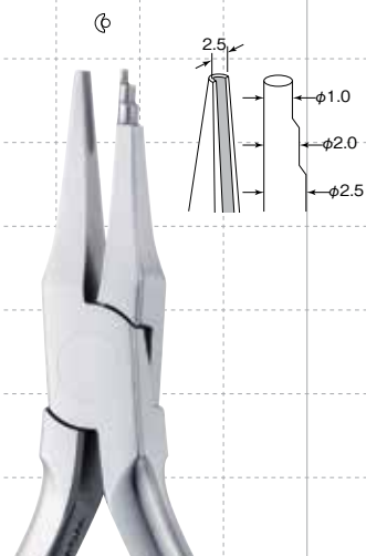
▲ 60-304S オメガ ループ フォーミング プライヤー OMEGA LOOP FORMING PLIER CODE NO.63041 全長：約 132mm Wires up to.022" (0.55mm)
