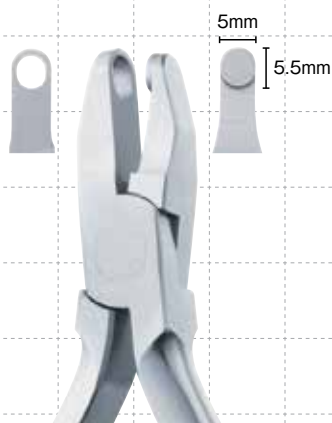
▲ 60-731 アライナー プライヤー ALIGNER PLIER Hole Punch CODE NO.67310 全長：約 125mm
