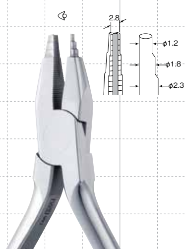
▲ 60-421 ループ フォーミング プライヤー 鶴見大型 LOOP FORMING PLIER OLD TYPE CODE NO.64210 全長：約 125mm Wires up to.025" (0.6mm)
