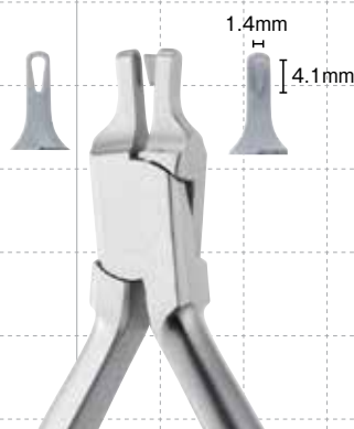
▲ 60-734 アライナー プライヤー ALIGNER PLIER Tear Drop CODE NO.67340 全長：約 118mm
