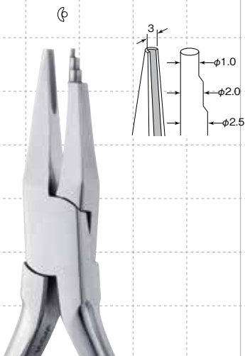
▲ 60-304 ツイード ループ フォーミング プライヤー TWEED LOOP FORMING PLIER CODE NO.63040 全長：約 131mm Wires up to.022" (0.55mm)
