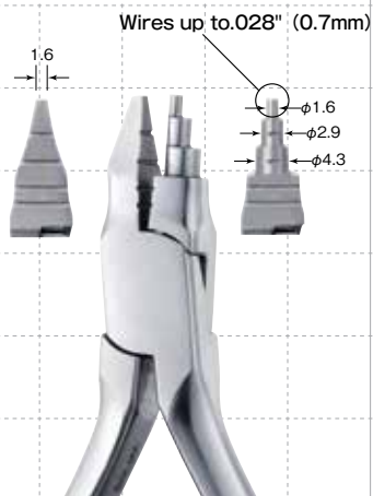
▲ 60-074 ヤング プライヤー YOUNG PLIER CODE NO.60740 全長：約 120mm Wires up to.028"~.040" (0.7~1.0mm)
